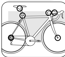
Mögliche Positionen von Schnellspannern, Steckachsen und Verschraubungen
