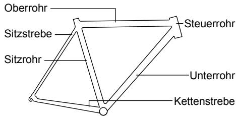
Gemuffter Stahlrahmen
