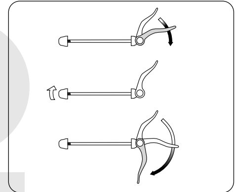
Einstellmutter lockern
